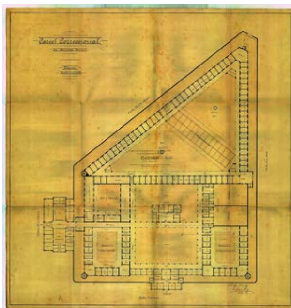
Fig.4- Proyecto de Cárcel Correccional. Planta. Autor: Enrique Aberg. 1883. Documento perteneciente al archivo del Centro de Documentación e Investigación de la Arquitectura Pública –CEDIAP- del CDI del Ministerio de Hacienda y Finanzas Públicas.
